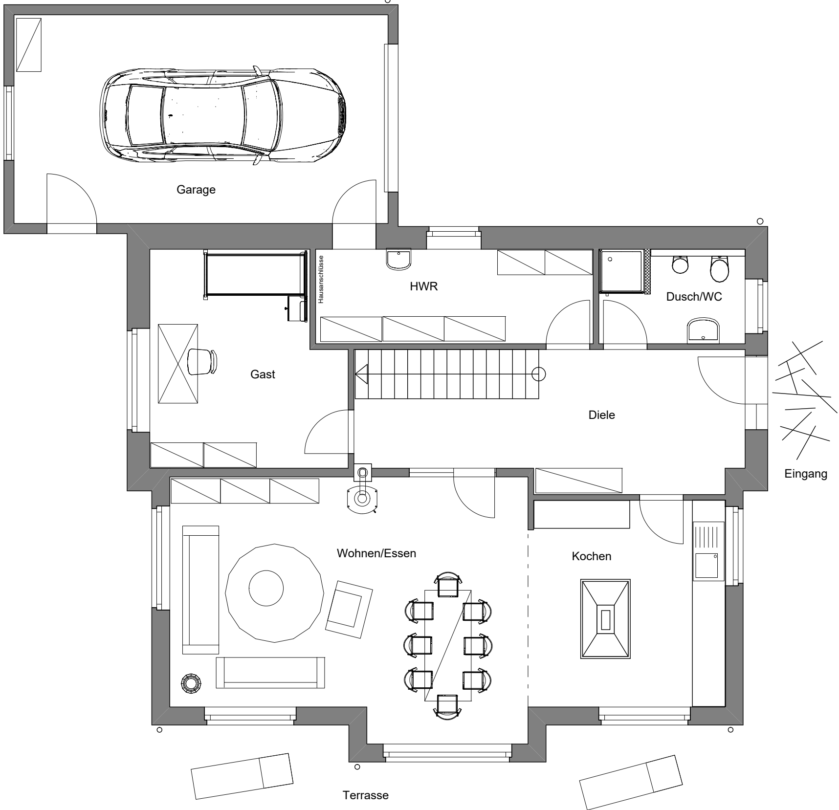
Wohngrundfläche Erdgeschoss: ca. 106,00 m 2
